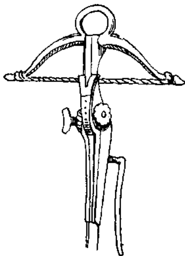
Fig. 79. - Balestra a ruota di ringranaggio del secolo XV (Race d'Ambras).
