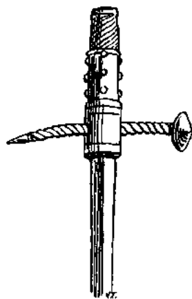
Fig. 418. - Fornamento di uno stocco da bastone, seconda metà secolo XVI.
